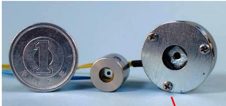
超小形無励磁作動 ブレーキ（丸形）
